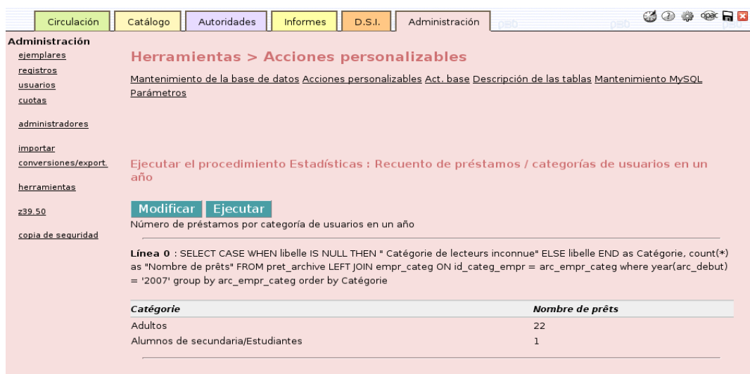
Figura 7.3: Resultado de ejecutar un procedimiento.
