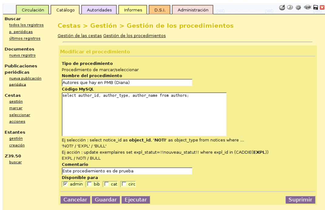
Figura 5.21: Modificar un procedimiento.
