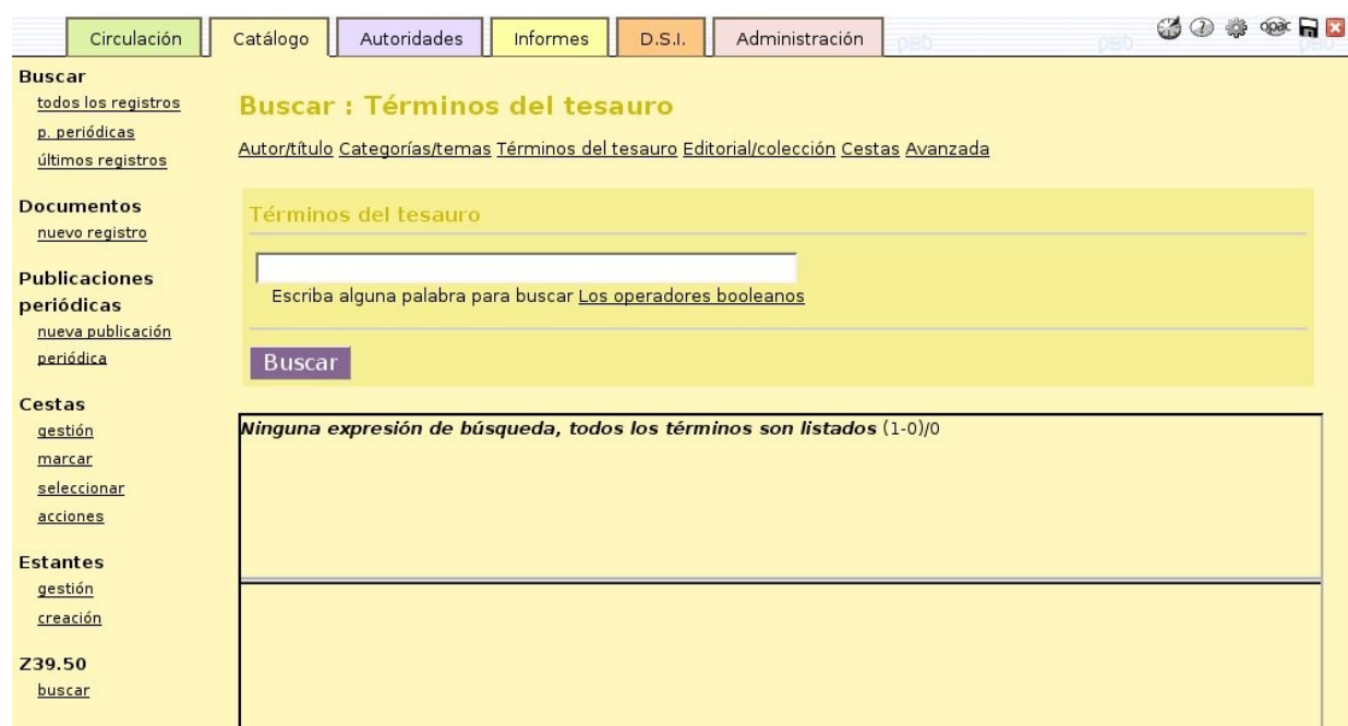
Figura 5.2: Pantalla de búsqueda de términos del tesoro.
