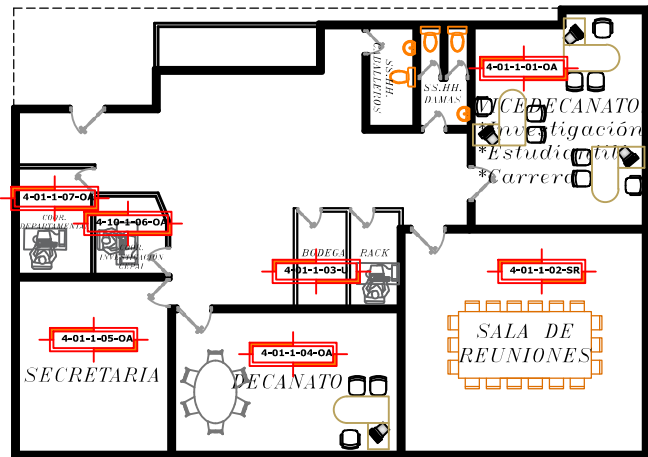
PLANTA BAJA ESC: 1/50 AREA=215.50m 2
