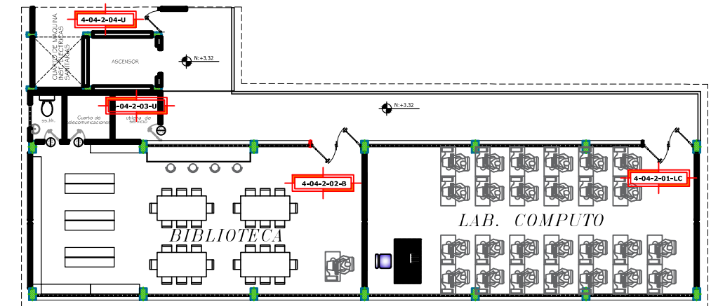
1ER PLANTA ALTA
