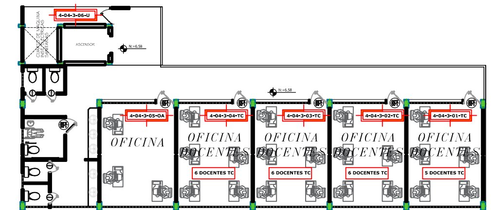
2DA PLANTA ALTA
