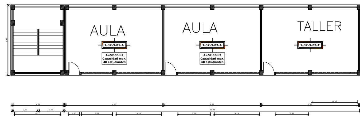
SEGUNDA PLANTA ALTA ESC: 1/100 AREA=207.05m²
