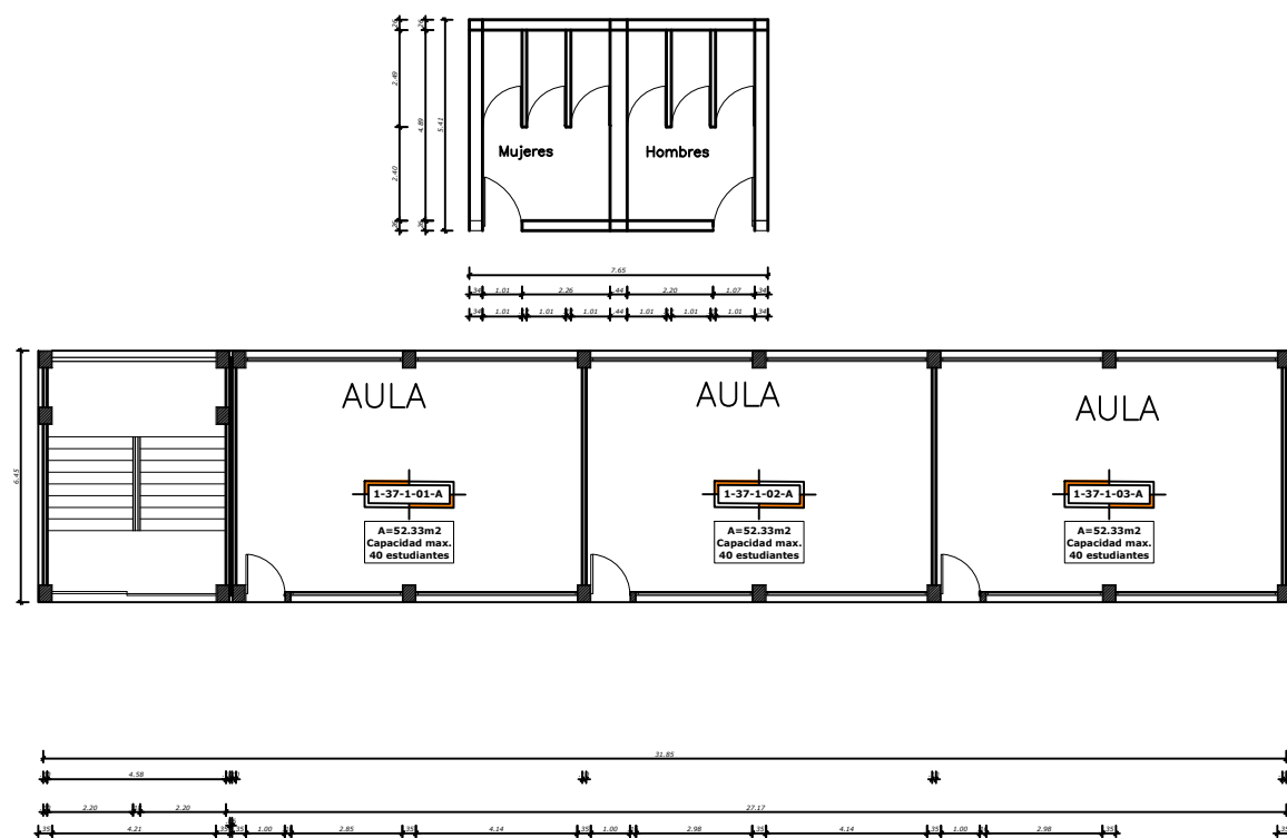
PLANTA BAJA Y BAÑOS ESC: 1/100 AREA=248.39m²
