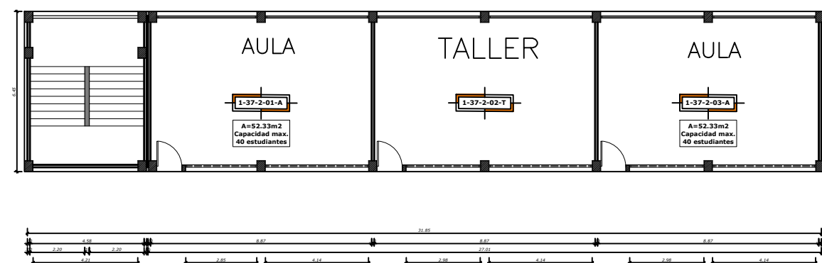
PRIMERA PLANTA ALTA ESC: 1/100 AREA=207.05m²
