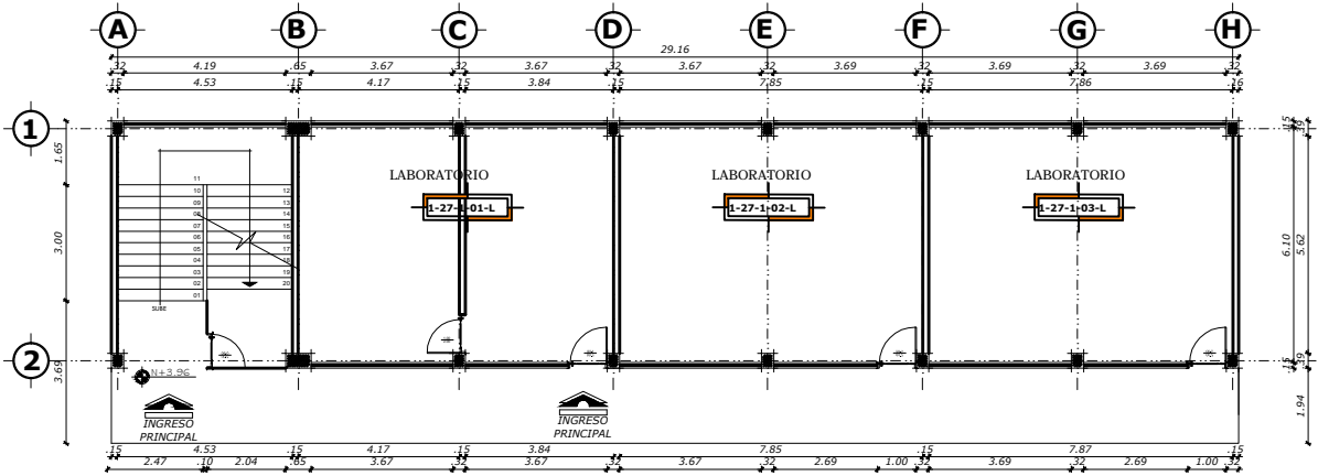
PLANTA BAJA ESC: 1/100 AREA=243.20m 2
