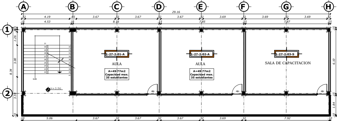
PRIMERA PLANTA ALTA ESC: 1/100 AREA=243.20m 2
