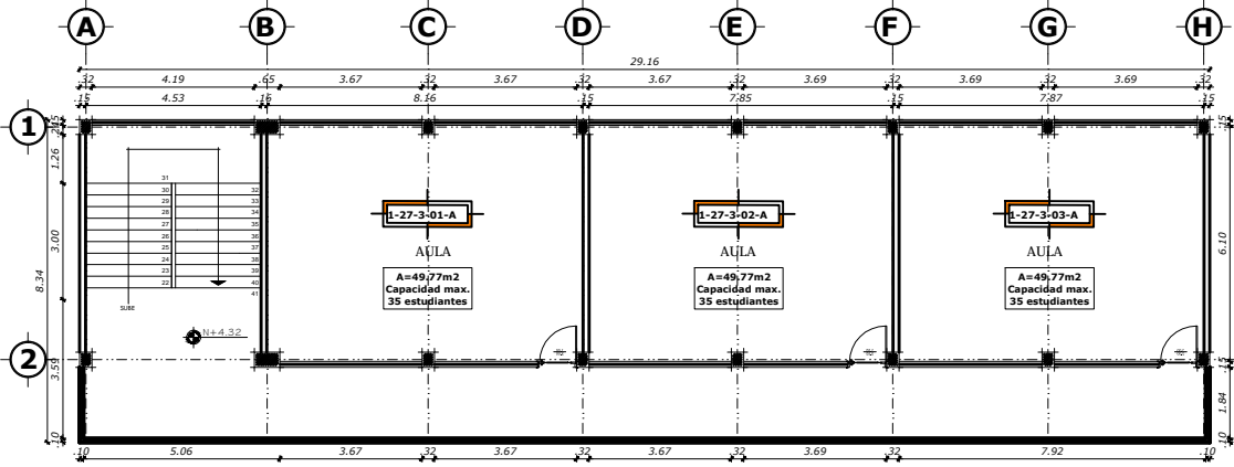
SEGUNDA PLANTA ALTA ESC: 1/100 AREA=243.20m 2
